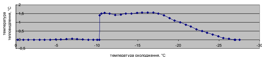
Рис. 1. Екзотерма льодоутворення в тканинах вишні сорту Подбельська
